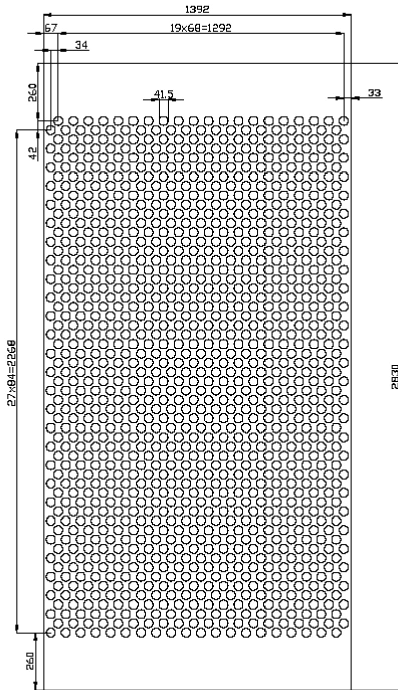
Raspored rupa na manjoj nosećoj ploči \delta=20\text{mm} crtaž broj 18-04-16b
