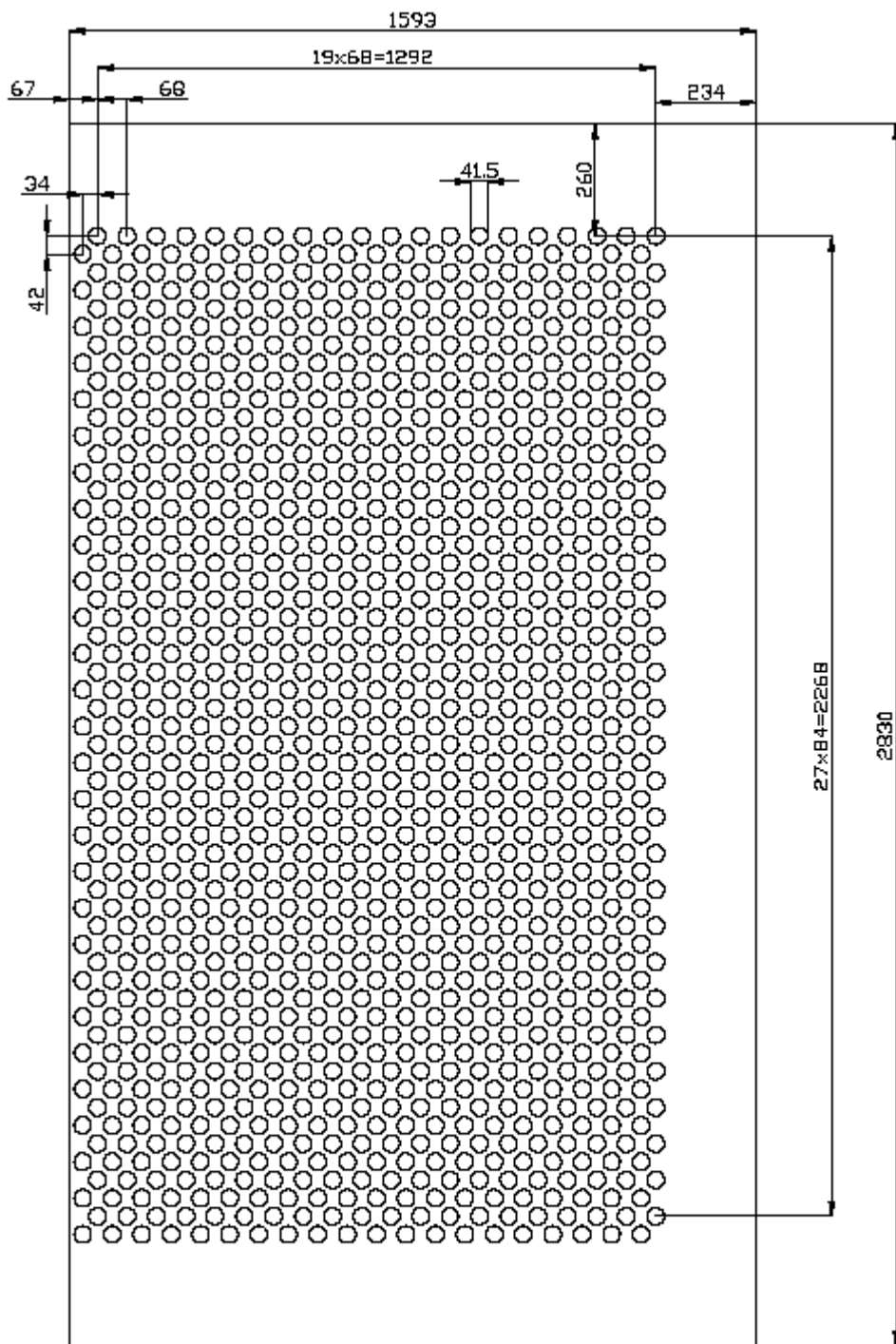
Raspored rupa na većoj nosećoj ploči \delta=20\text{mm} crtež broj 18-04-16a
